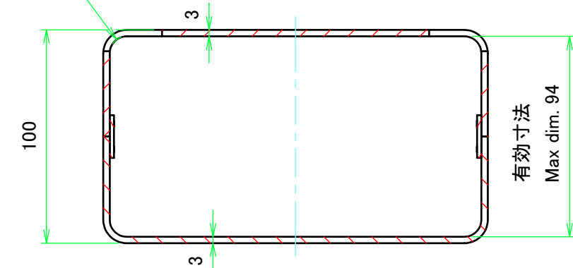
D-D (1:2.5)
