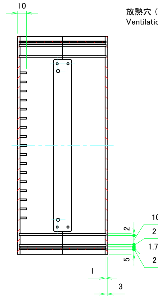
B-B (1:2.5)
