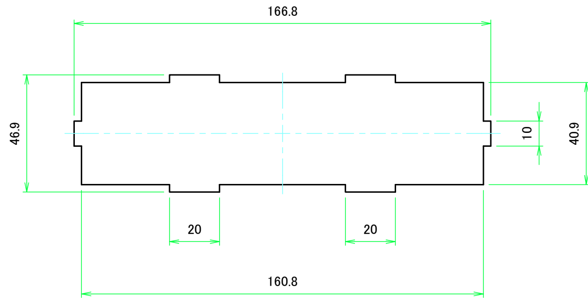
Dパネル1表面 / D Panel 1 Frontside
