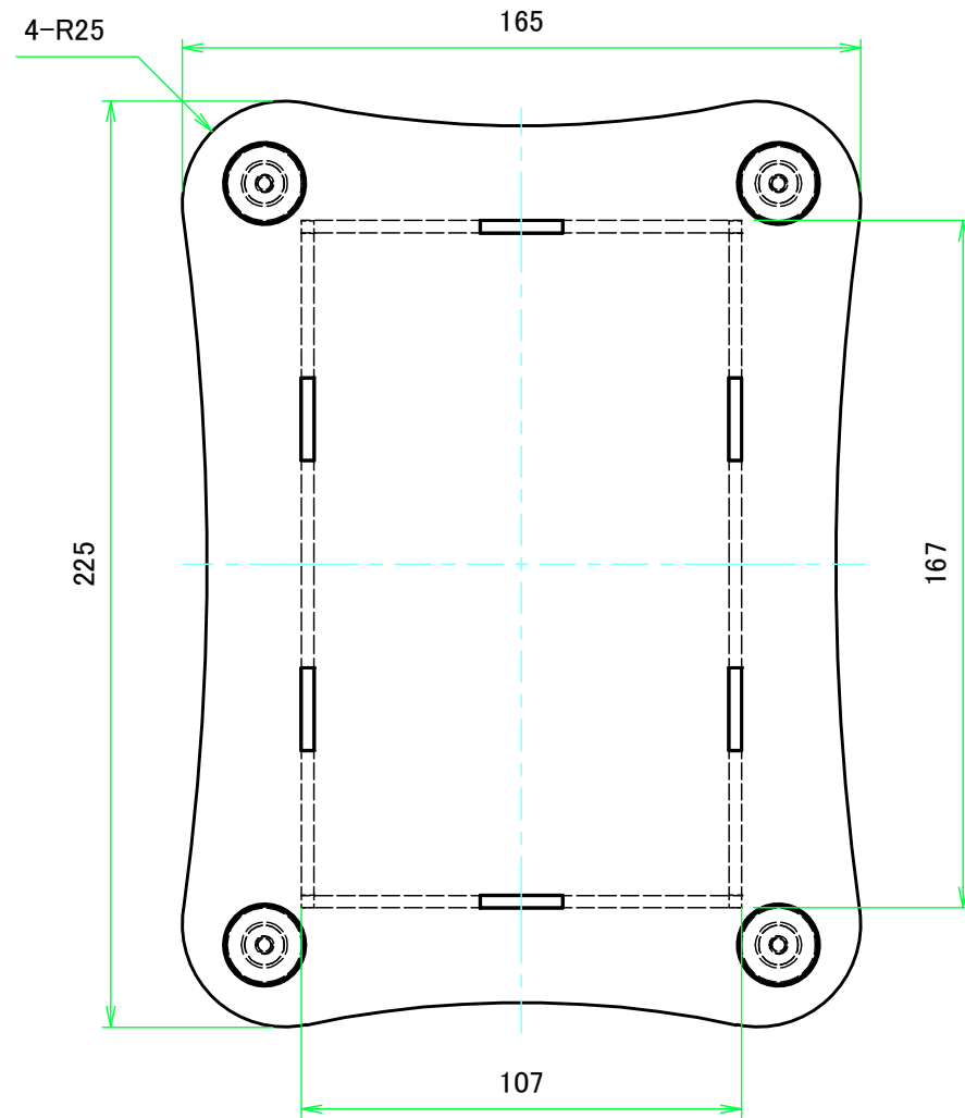
上カバー / Top cover
