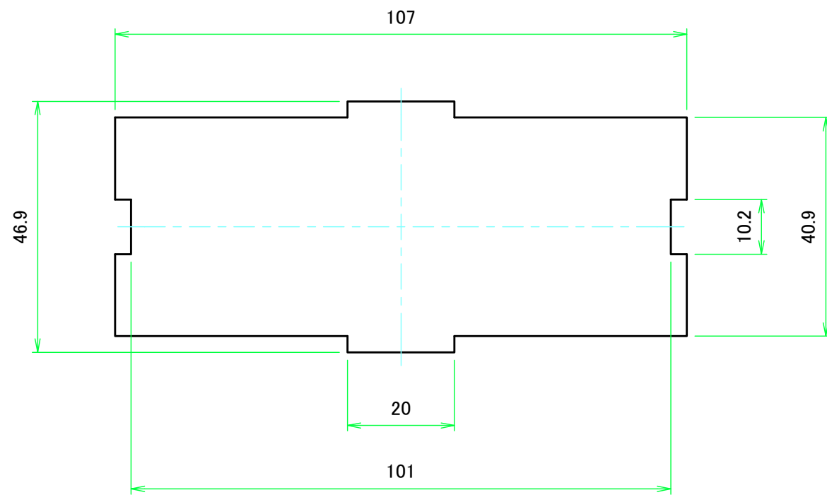
Wパネル1表面 / W Panel 1 Frontside
