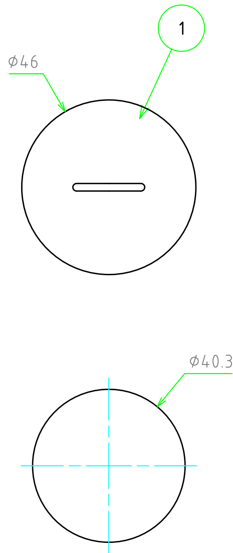
取付穴寸法
