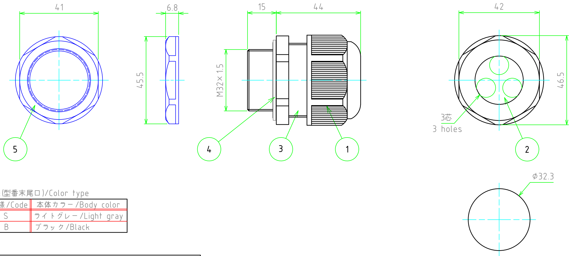
取付穴寸法 /Mounting hole dimensions
