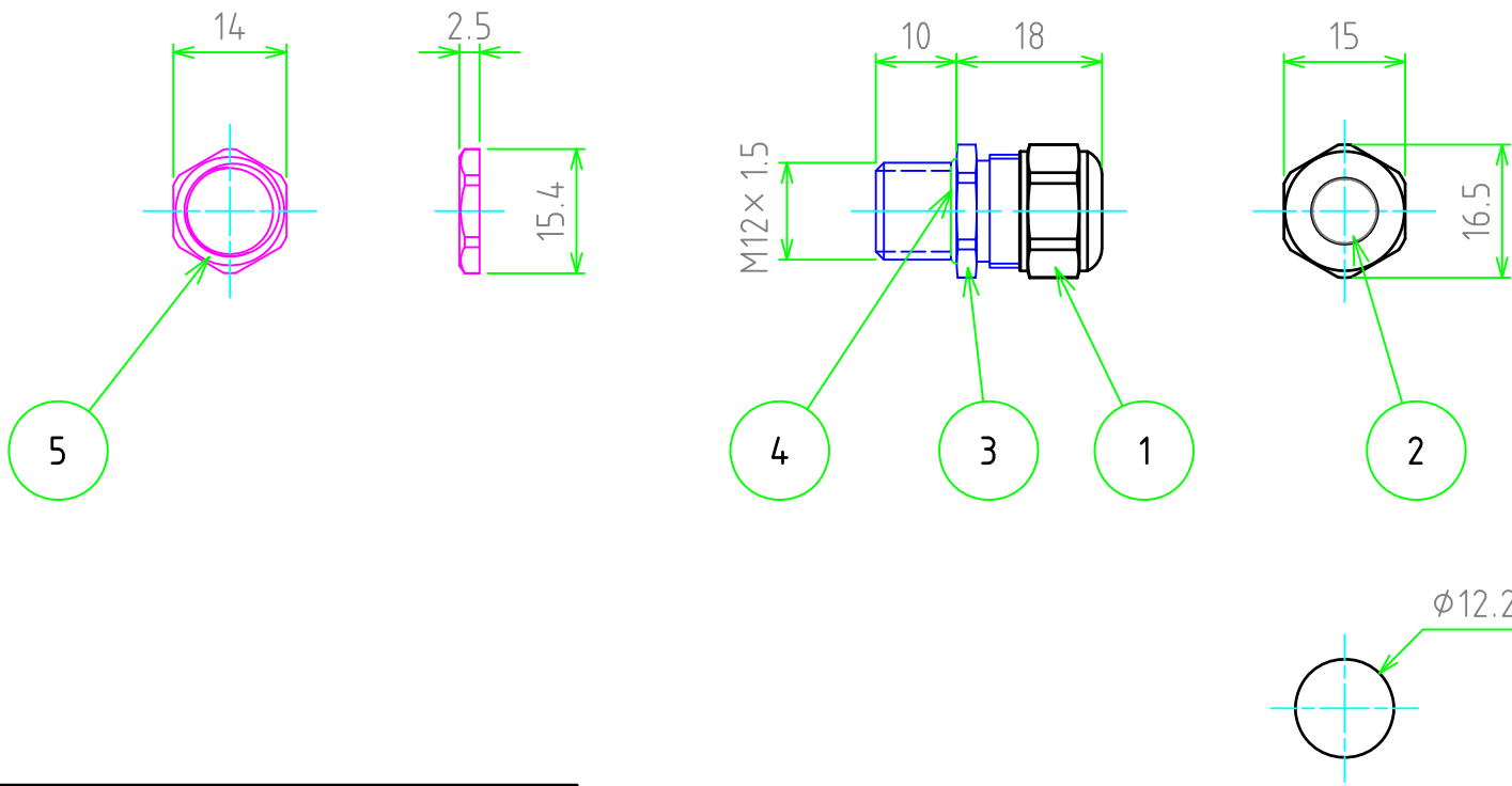
取付穴寸法 / Mounting hole dimensions
