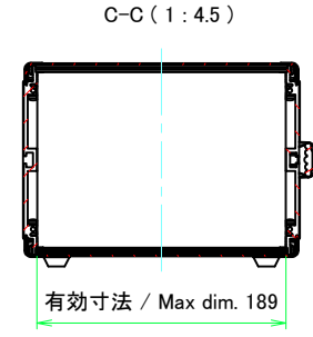
リアフレーム2 / Rear frame2
