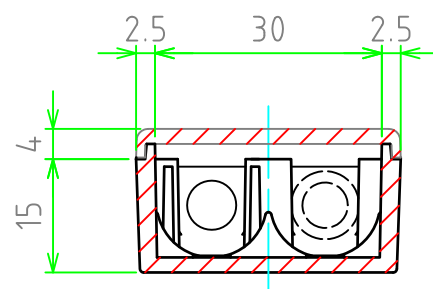
B-B断面図
