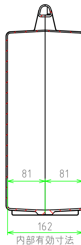
A-A 断面図
