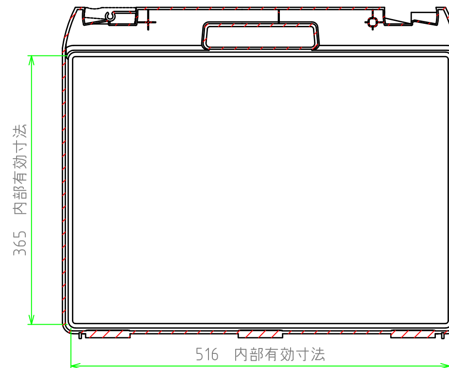
B-B 断面図
