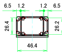
A-A (1:2.5)
