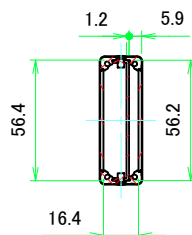
A-A (1:2.5)
