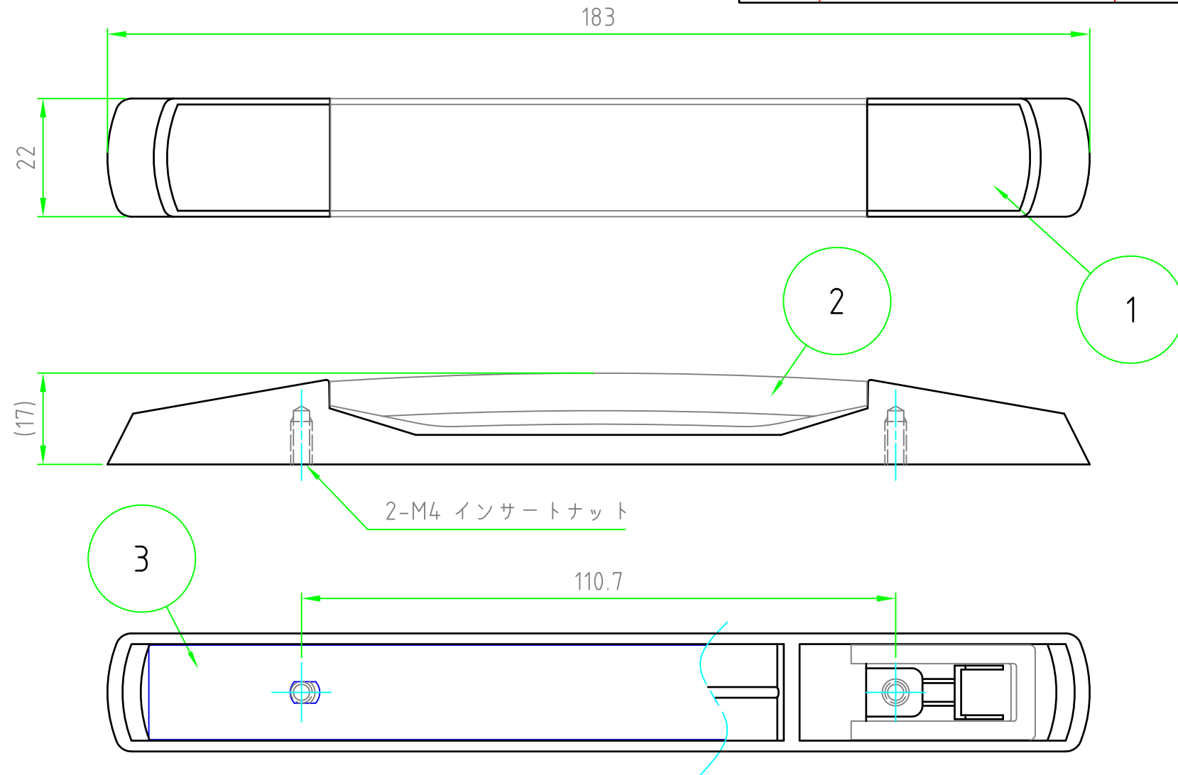
取付穴寸法図
