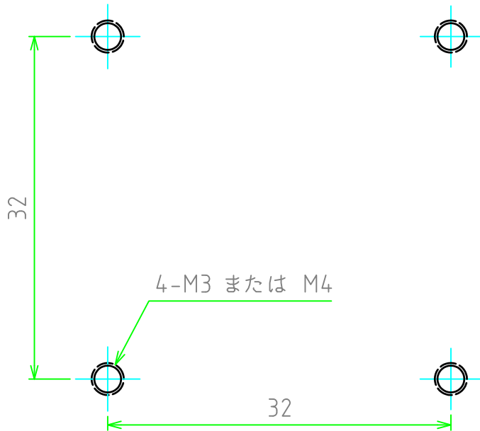
取付穴寸法
