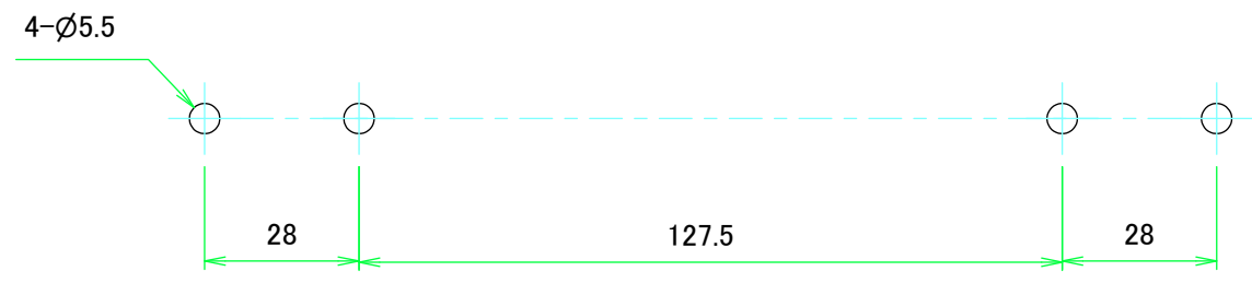
取付寸法図 / Mounting dimensions
