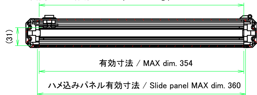
開閉パネル有効寸法 / Open-closing panel MAX dim. 354
