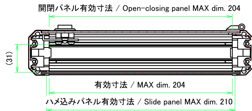
A-A (1:2.5)
