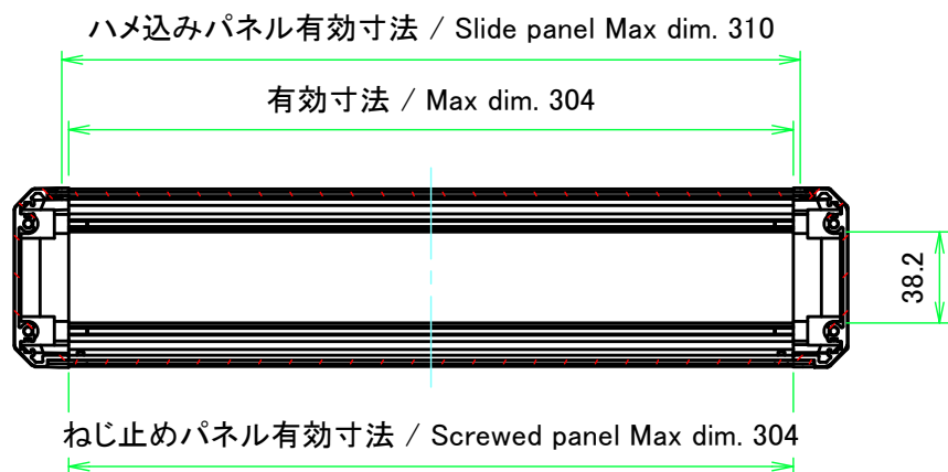
A-A (1:3.5)
