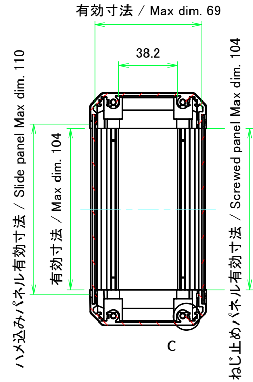
B-B (1:2.5)
