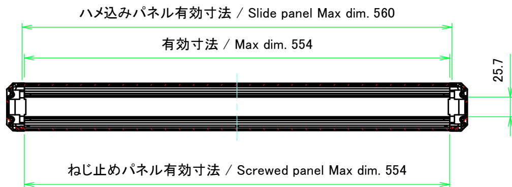
A-A (1:5)
