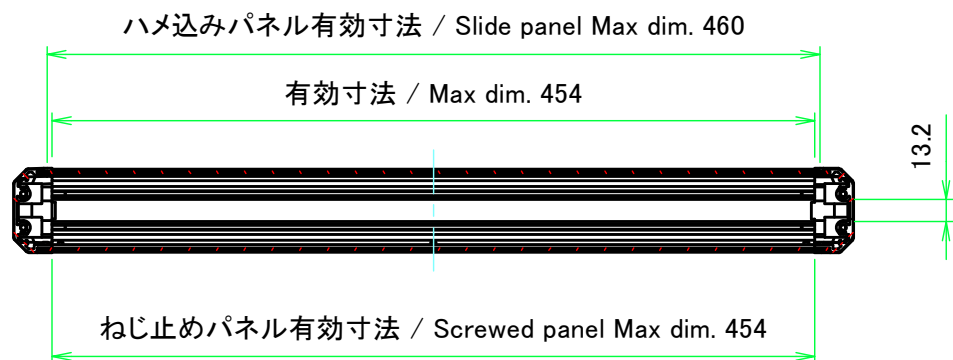
A-A (1:4.5)
