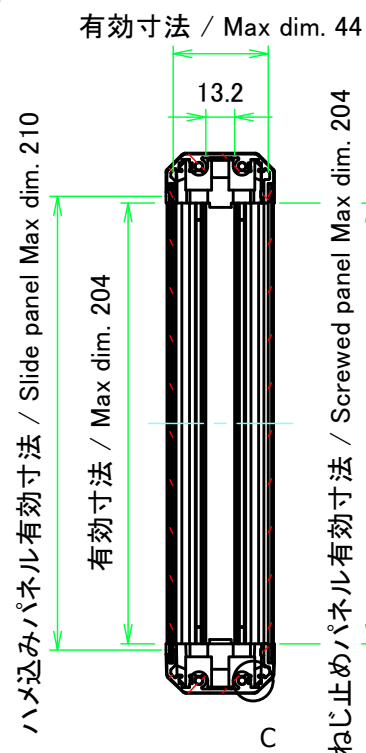
B-B (1:3.5)
