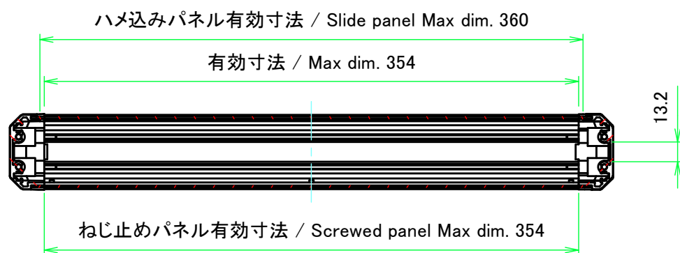
A-A (1:3.5)
