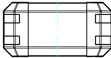
A-A (1:2) ハメ込みパネル有効寸法 / Slide panel Max dim. 60
