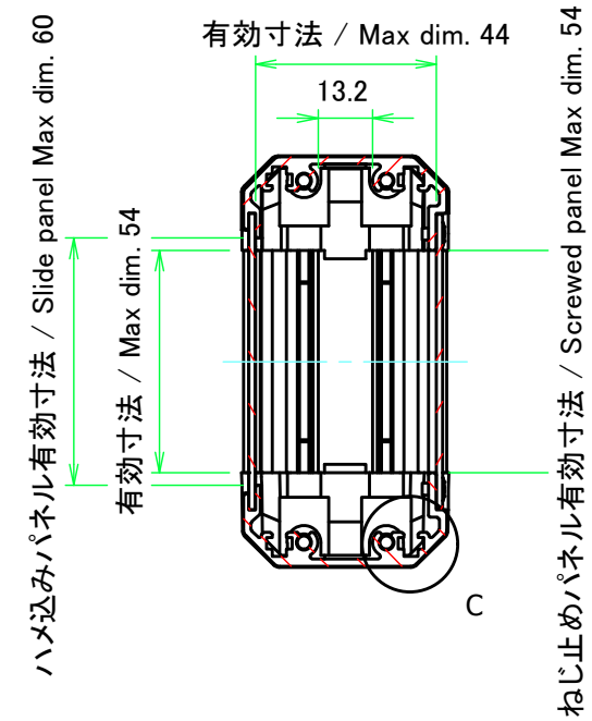
B-B (1:2)
