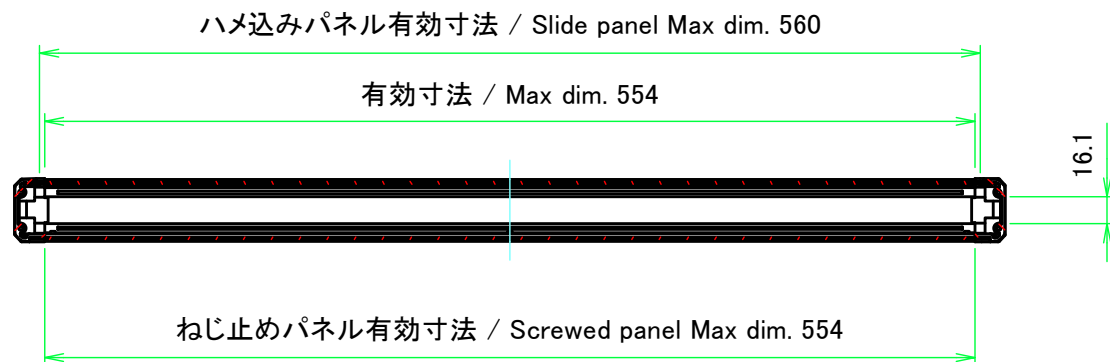
A-A (1:4.5)
