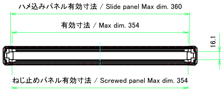
A-A (1:4)
