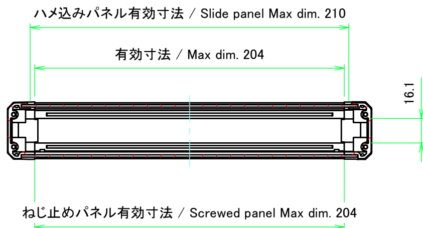
A-A (1:2.5)
