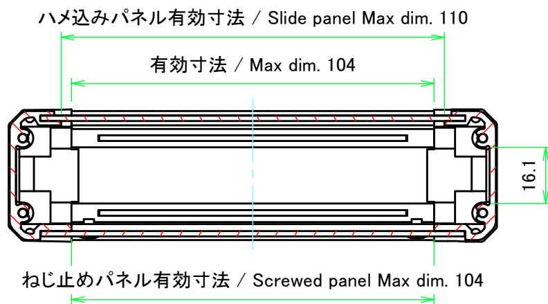
A-A (1:1.5)
