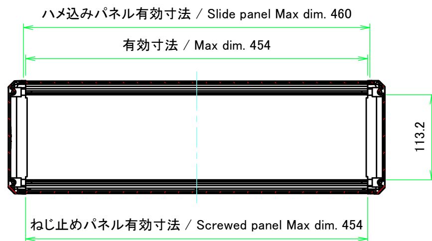
A-A (1:5)
