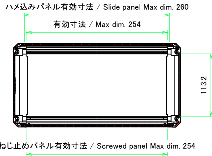
A-A (1:4)
