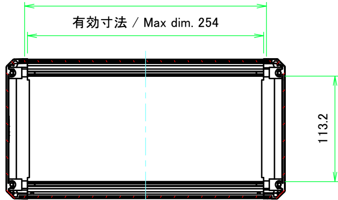
ハメ込みパネル有効寸法 / Slide panel Max dim. 260
