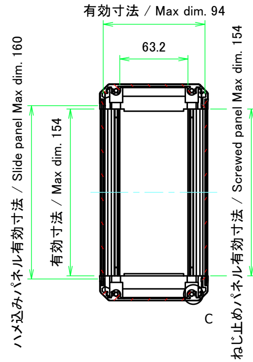
B-B (1:3.5)
