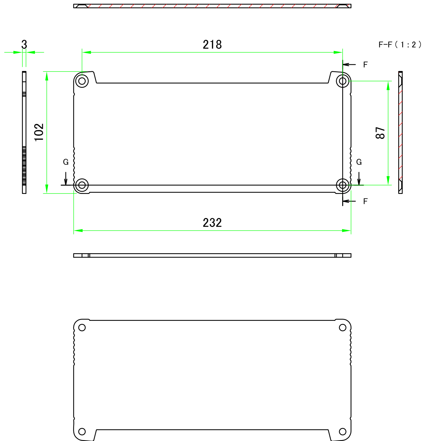
G-G (1:2)
