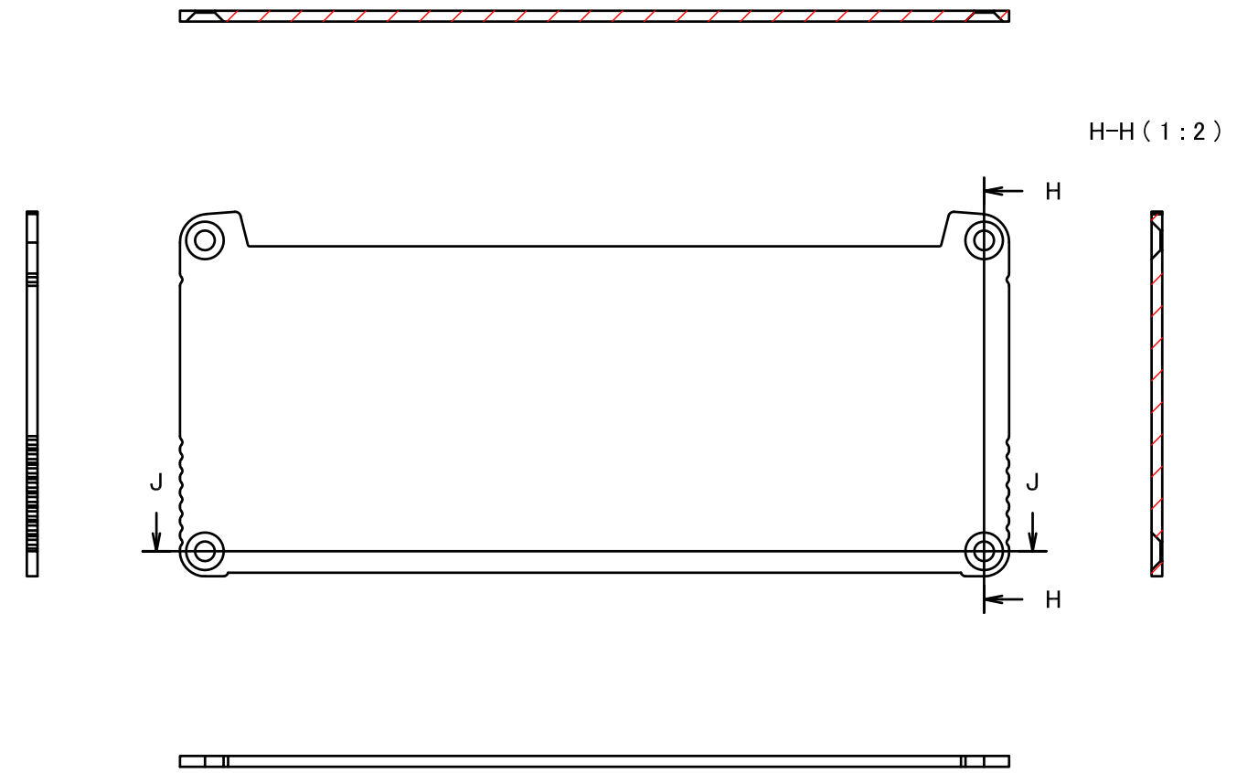
J-J (1:2)
