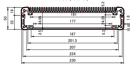
A-A (1:4)
