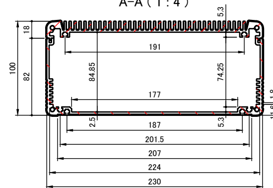
A-A (1:4)
