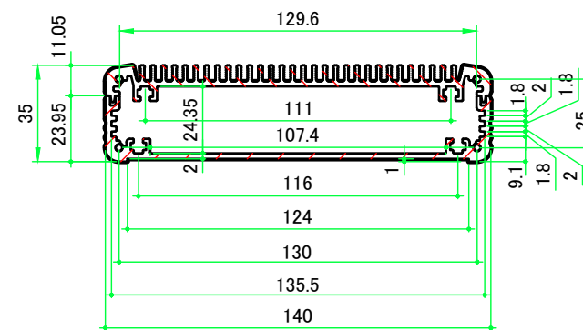
A-A (1:2.5)
