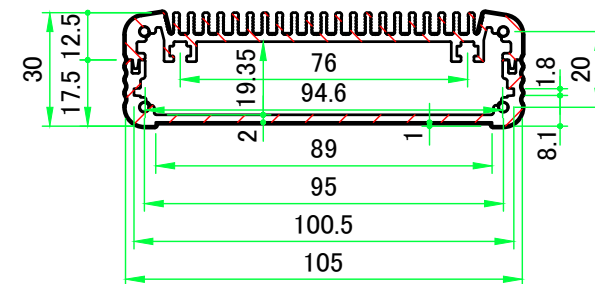
A-A (1:2)
