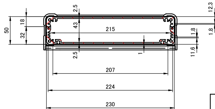
A-A (1:4)
