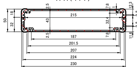
A-A (1:4)
