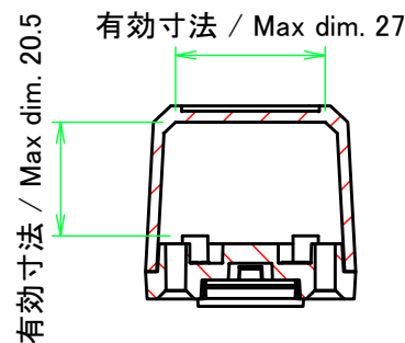
A-A ( 1:1.5 )
