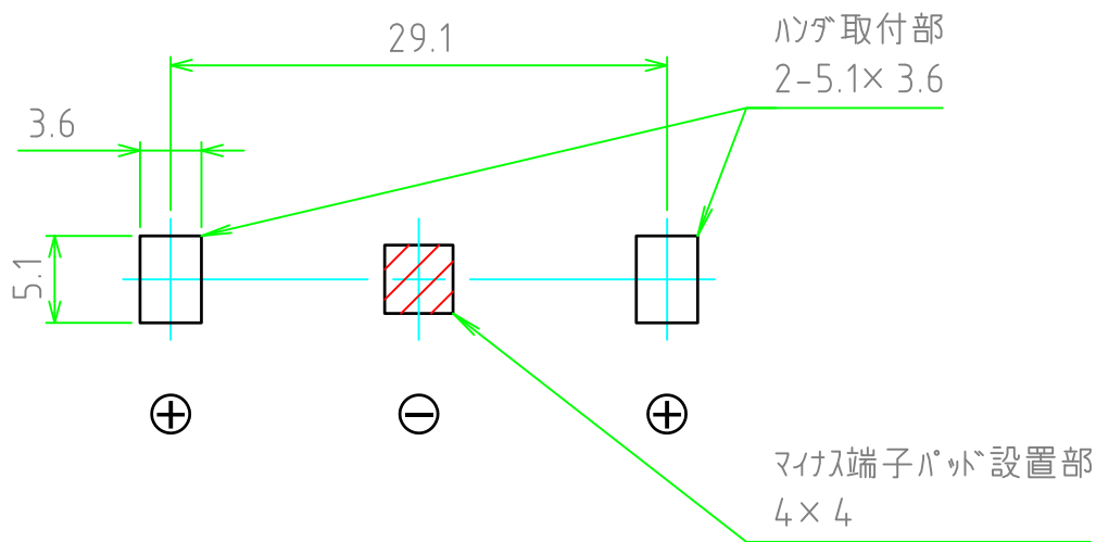
基板実装図
