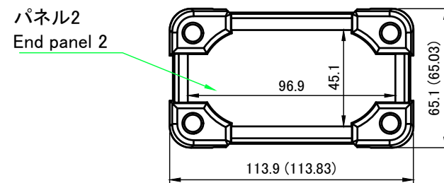
A-A (1:2.5)
