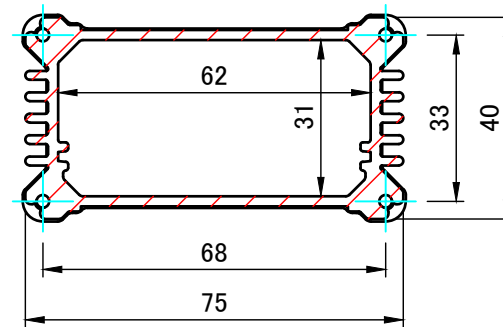
A-A (1:1.5)
